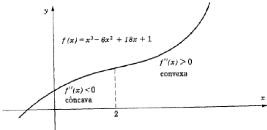
Figura 18. Función Cóncava y Convexa
