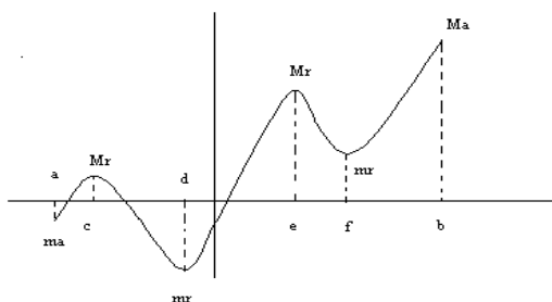
Figura 15. Curva de Máximo y Mínimo Relativo
