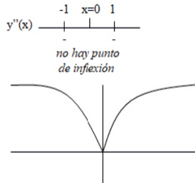
Figura 24. Sin punto de Inflexión
