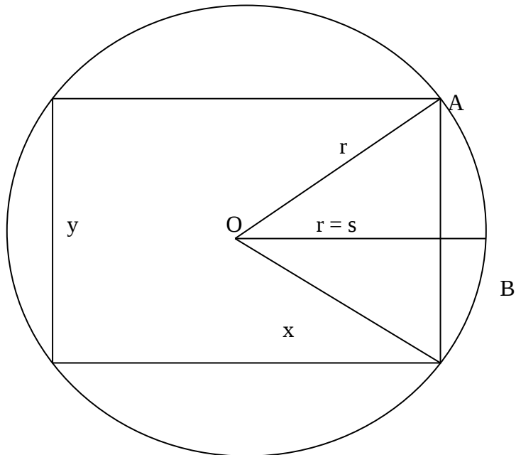
Figura 29. Rectángulo Inscrito en la Circunferencia
