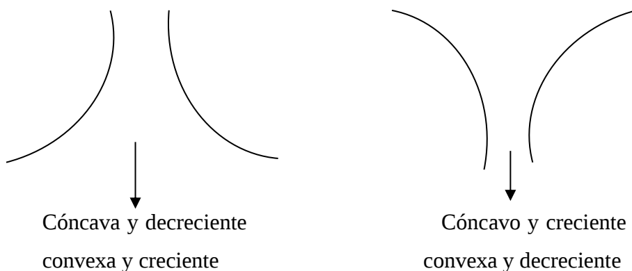
Figura 19. Concavidad y Convexidad (Leithold, L. , 1992)
