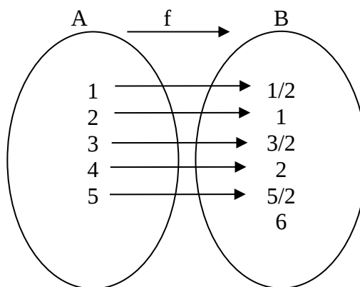
Figura 1. Dominio y Recorrido
