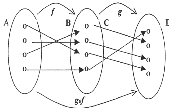
Figura 2. Composición de Funciones
