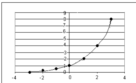
Figura 3. Función f(x) = 2^x
