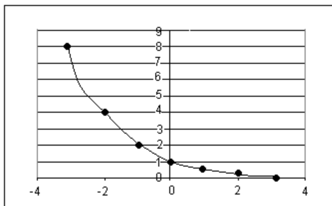
Figura 4. La función es decreciente.
