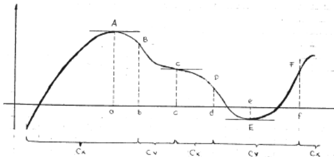
Figura 20. Puntos de Inflexión
